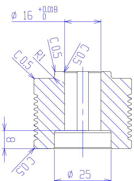
断面図 A-A スケール 1 : 1
